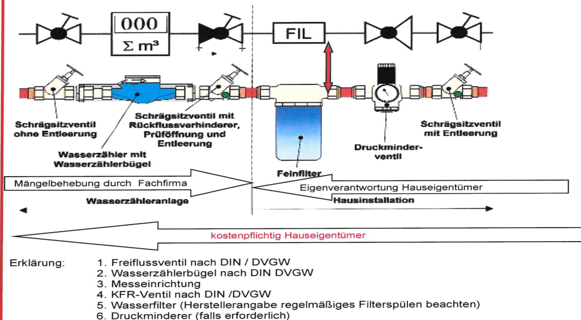
Schema einer korrekt installierten Wasserzähler-Anlage nach DIN 1988:
